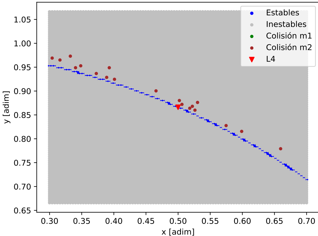
Mapa de estabilidad - 55_Cnc_55_Cnc_e
