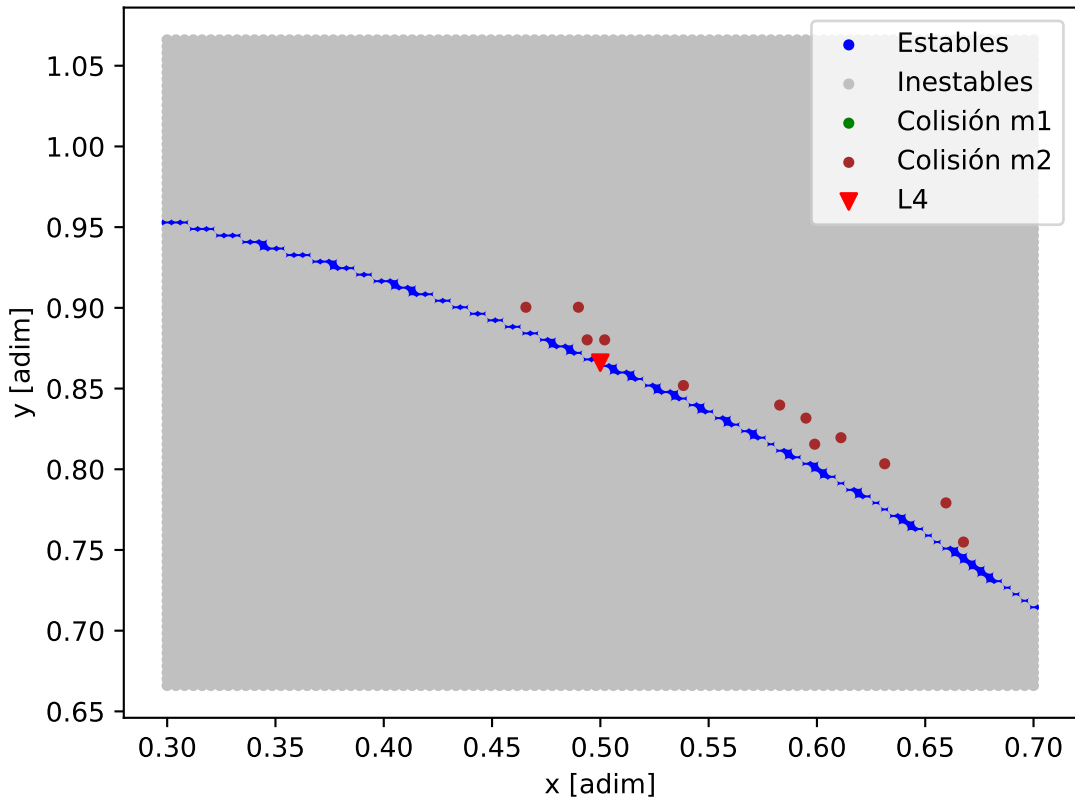
Mapa de estabilidad - EPIC_249893012_EPIC_249893012_d
