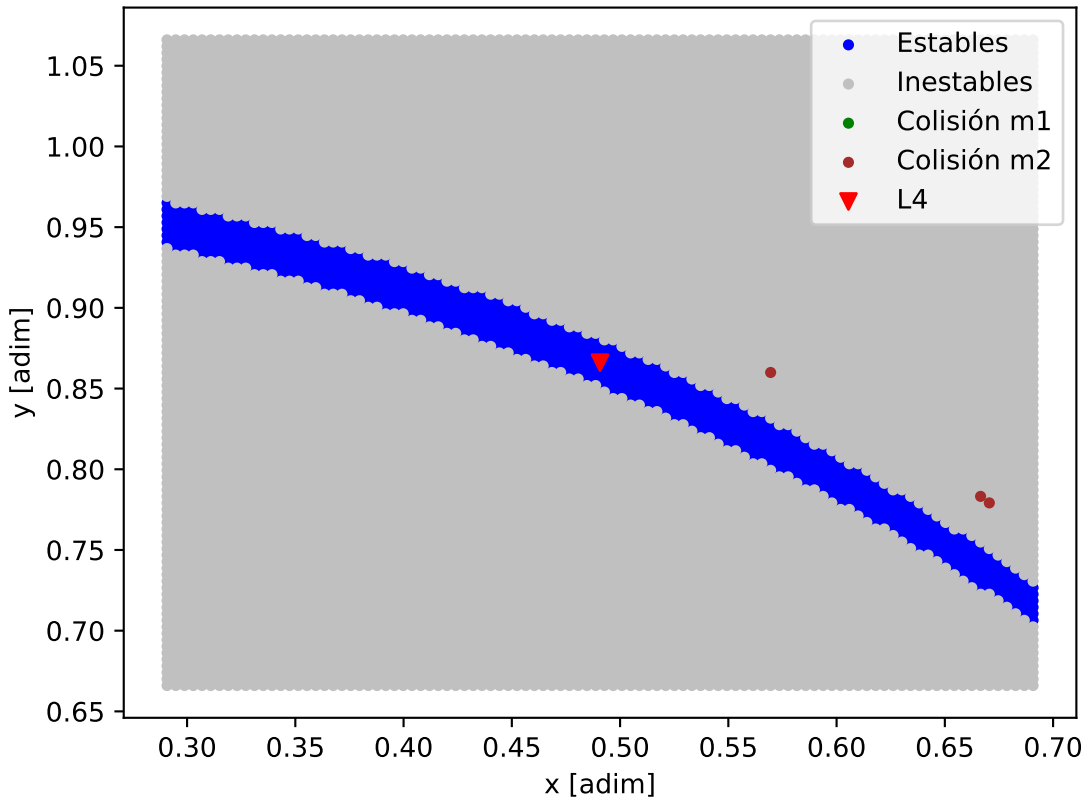
Mapa de estabilidad - HD_10180_HD_10180_d
