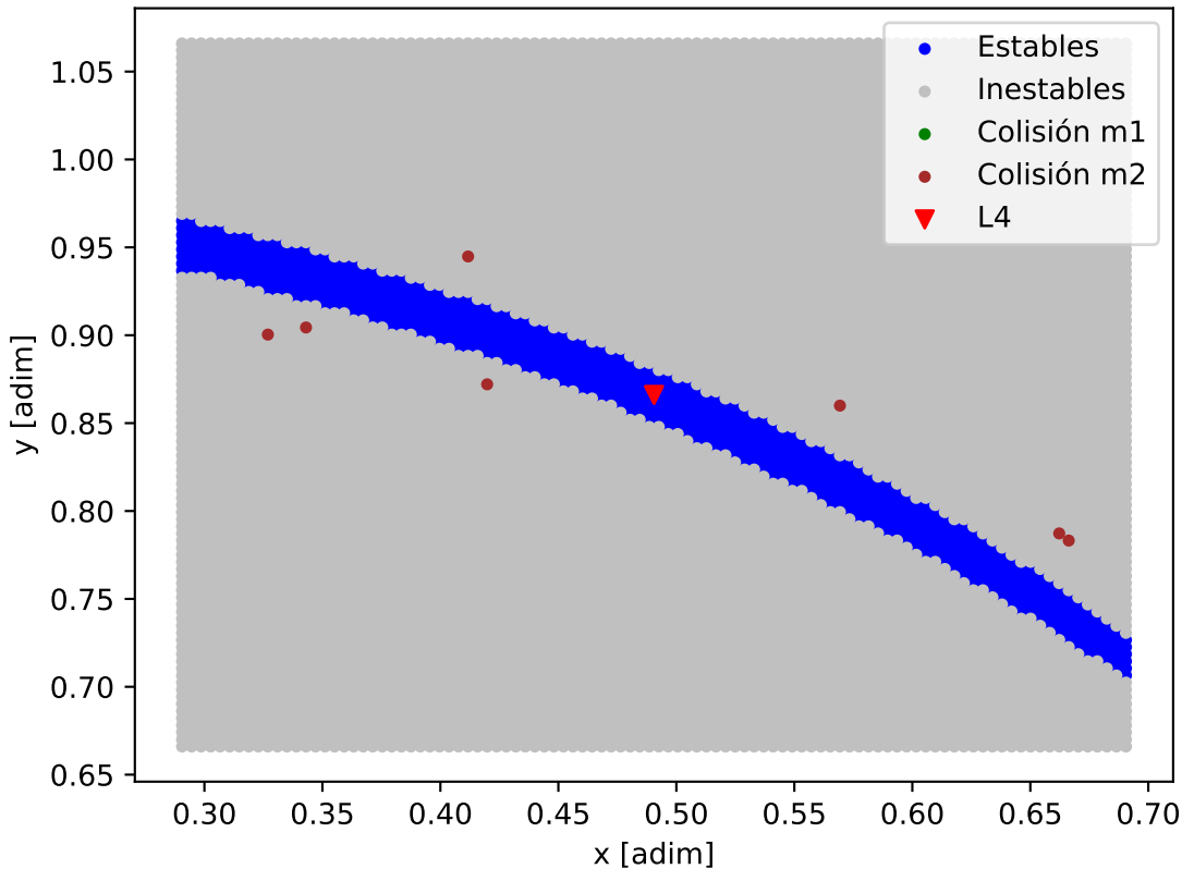
Mapa de estabilidad - HD_10180_HD_10180_g
