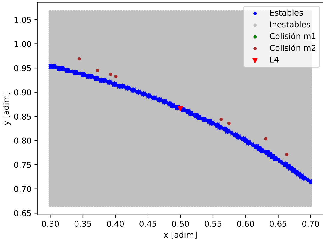
Mapa de estabilidad - HD_10180_HD_10180_h
