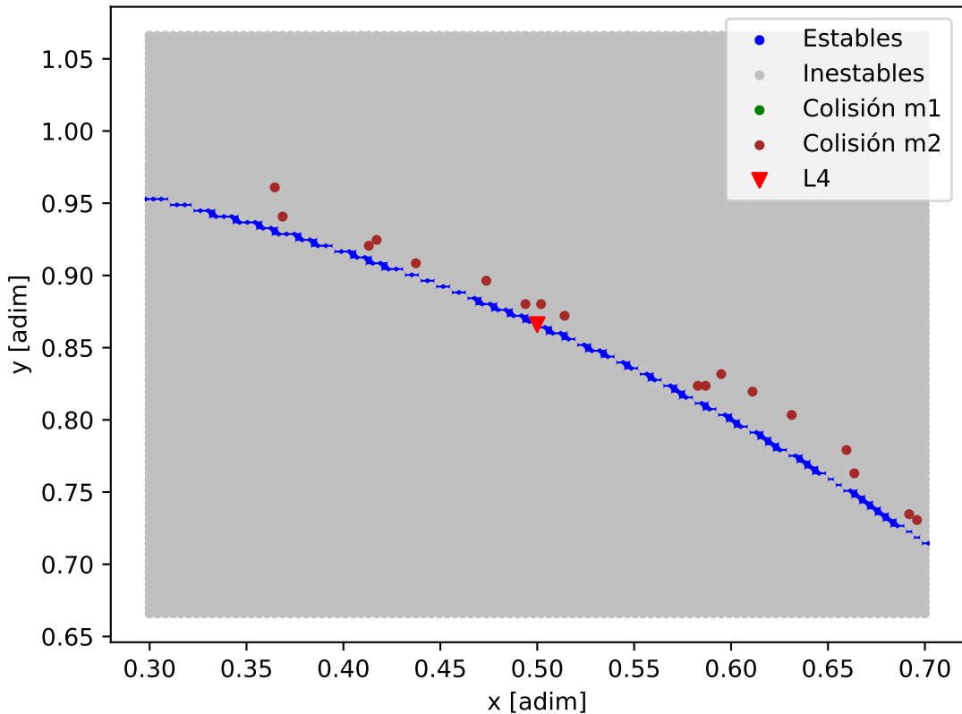
Mapa de estabilidad - HD_108236_HD_108236_e
