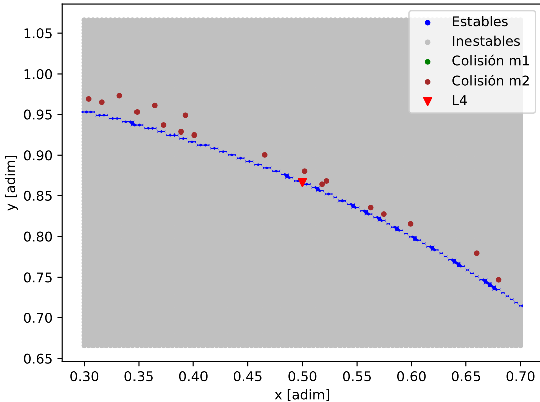
Mapa de estabilidad - HD_108236_TOI-1233.01
