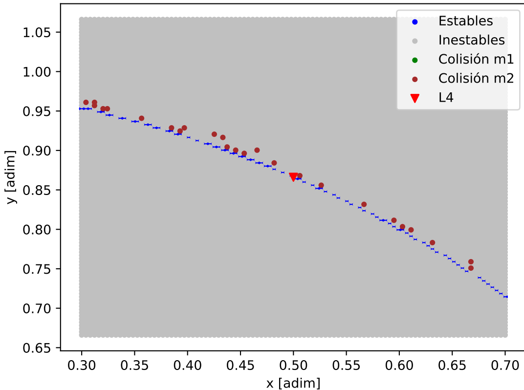
Mapa de estabilidad - HD_134606_HD_134606_e
