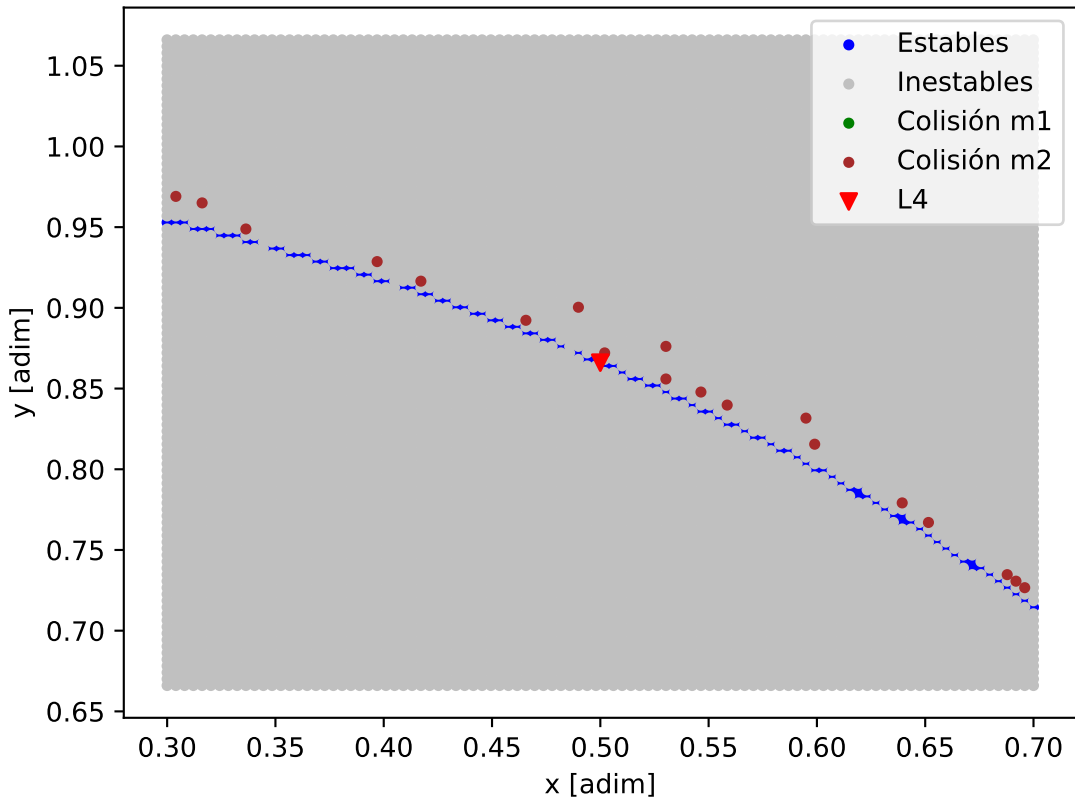
Mapa de estabilidad - HD_134606_HD_134606_f
