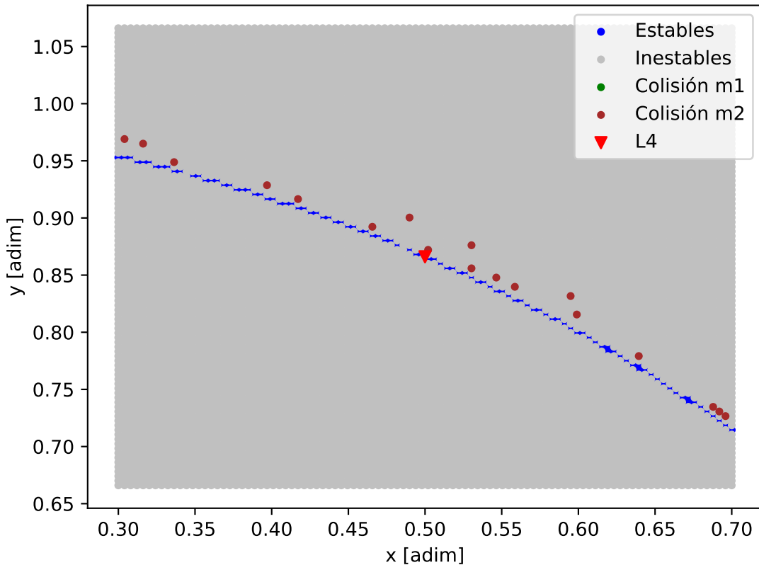
Mapa de estabilidad - HD_136352_HD_136352_b
