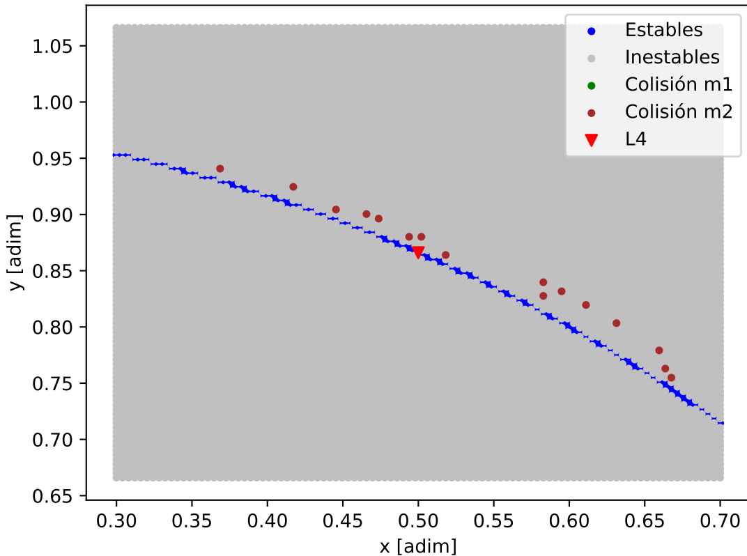
Mapa de estabilidad - HD_136352_HD_136352_d
