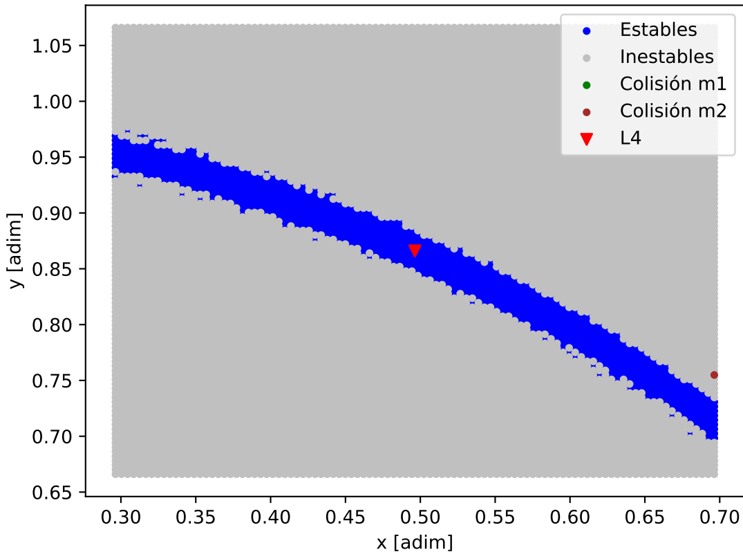
Mapa de estabilidad - HD_160691_HD_160691_b
