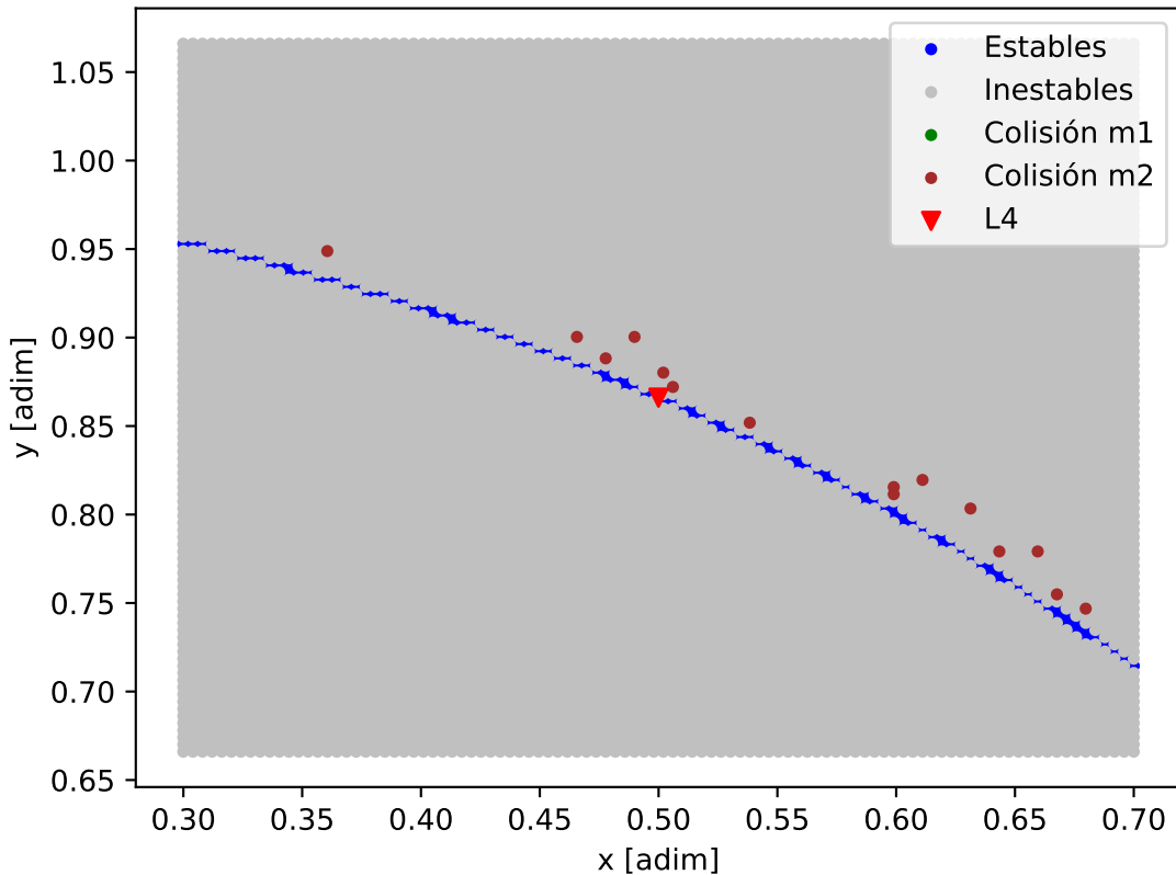
Mapa de estabilidad - HD_160691_HD_160691_d
