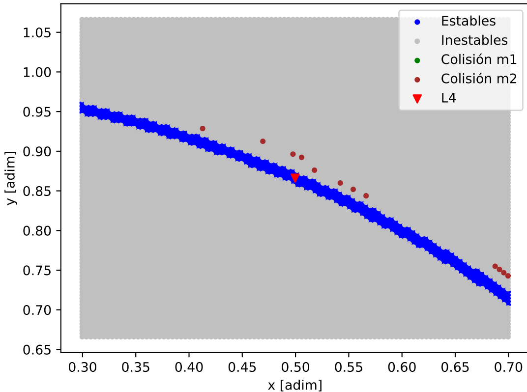
Mapa de estabilidad - HD_164922_HD_164922_b
