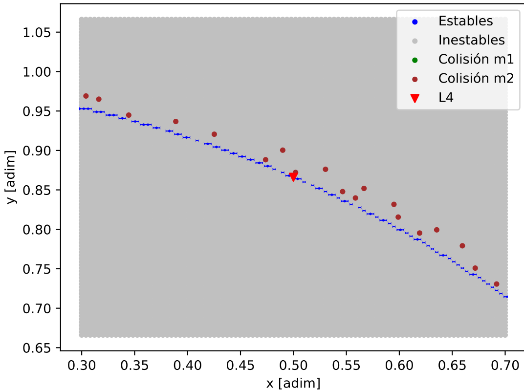
Mapa de estabilidad - HD_164922_HD_164922_d
