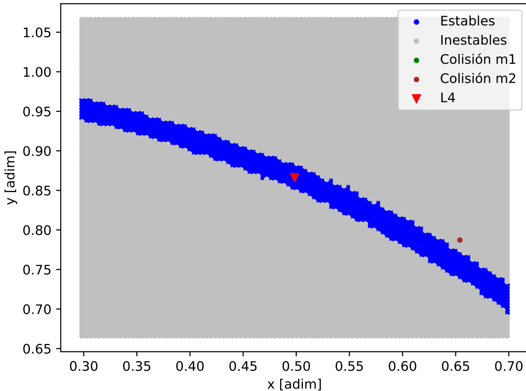
Mapa de estabilidad - HD_190360_HD_190360_b
