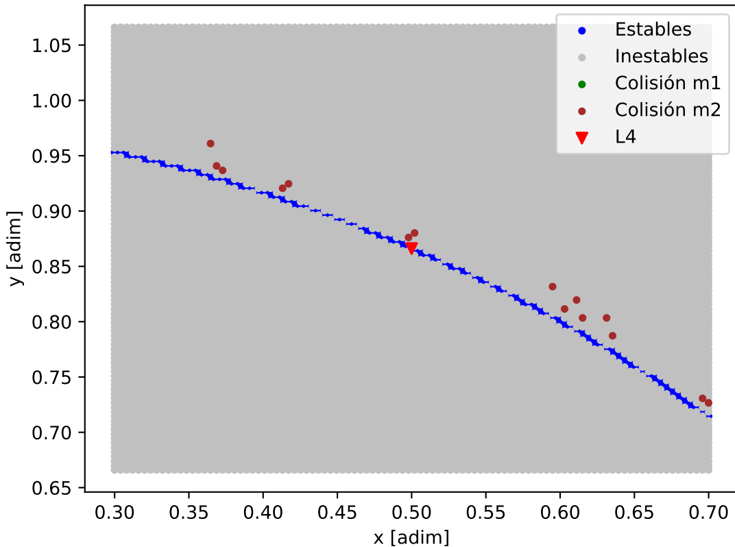
Mapa de estabilidad - HD_190360_HD_190360_d
