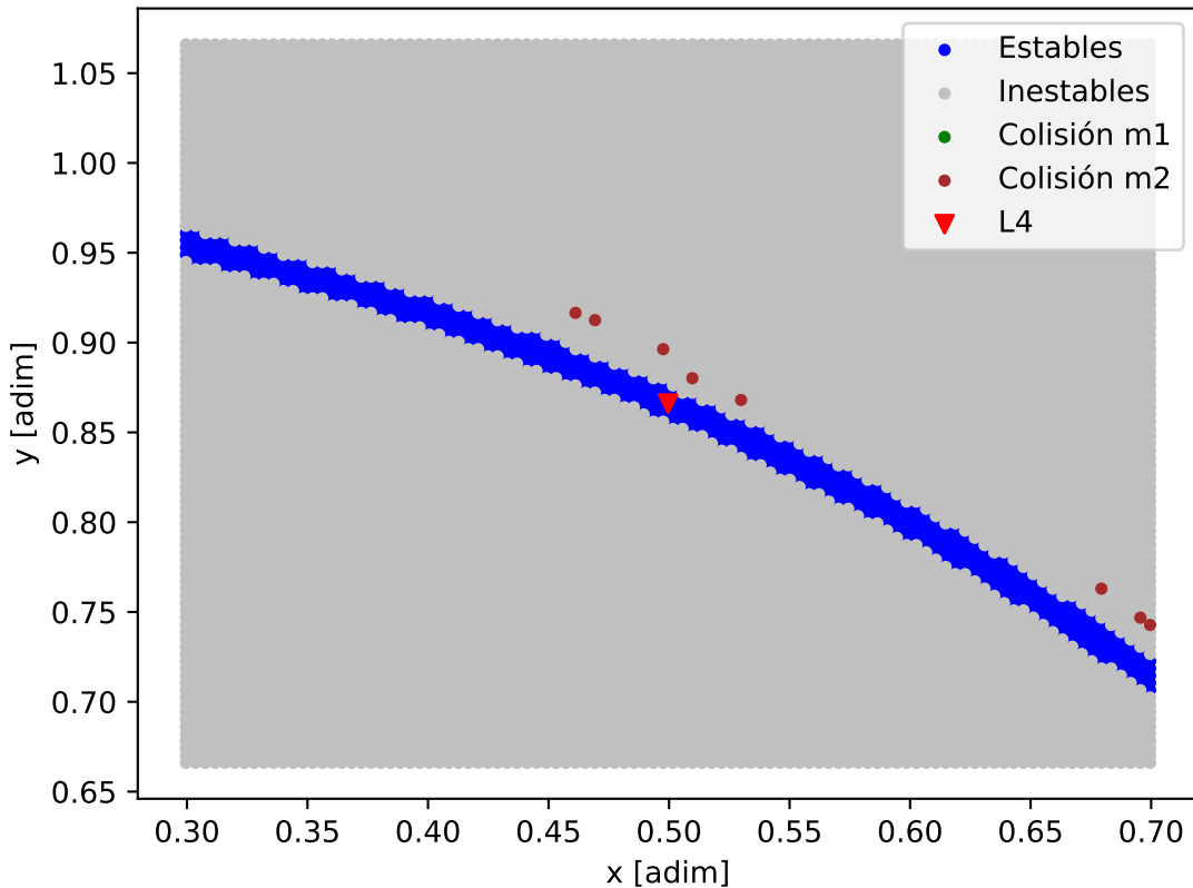
Mapa de estabilidad - HD_191939_HD_191939_e
