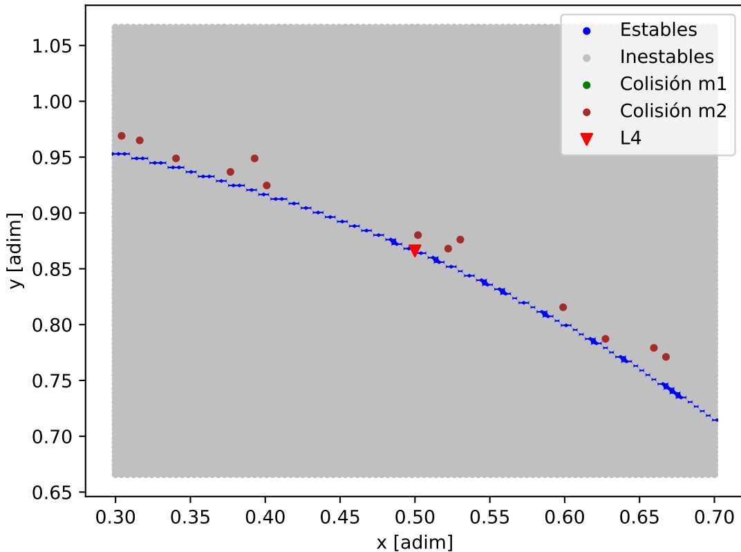
Mapa de estabilidad - HD_20794_HD_20794_f
