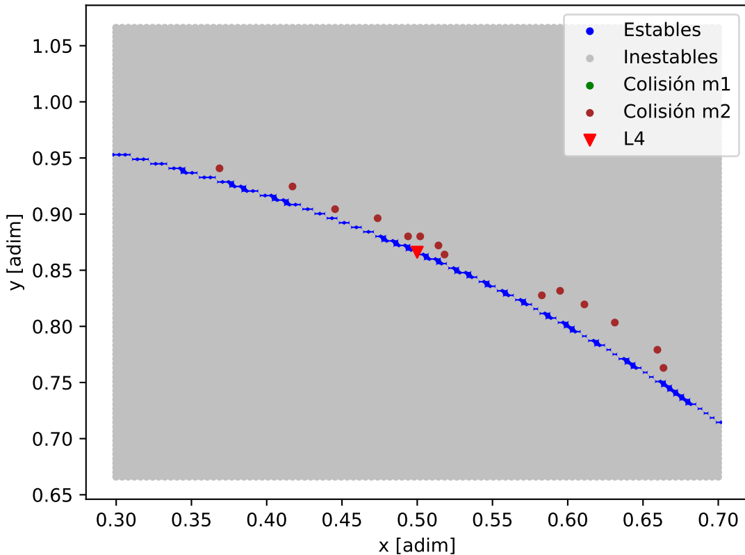
Mapa de estabilidad - HD_224018_HD_224018_c
