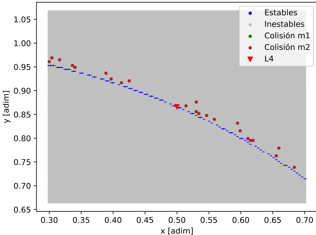
Mapa de estabilidad - HD_28471_HD_28471_b
