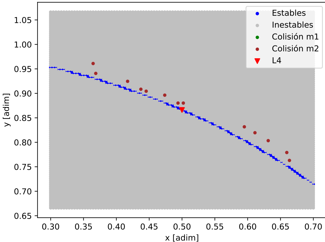
Mapa de estabilidad - HD_31527_HD_31527_b
