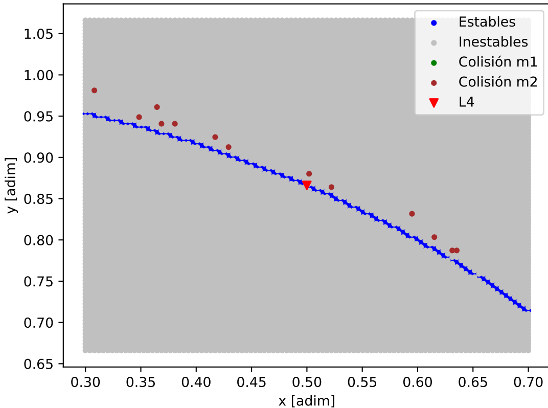
Mapa de estabilidad - HD_31527_HD_31527_c
