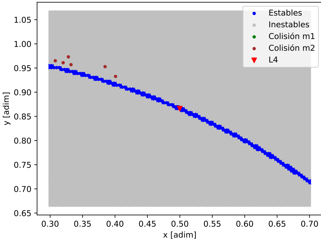
Mapa de estabilidad - HD_34445_HD_34445_c
