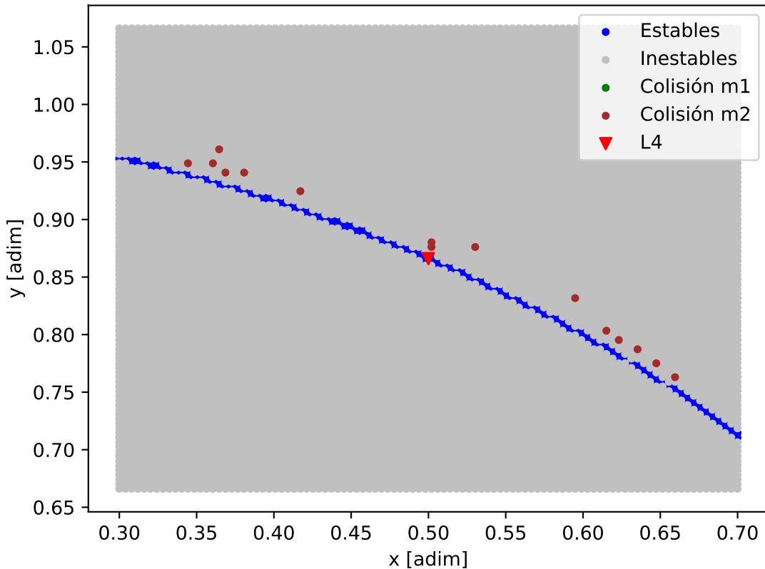
Mapa de estabilidad - HD_34445_HD_34445_e
