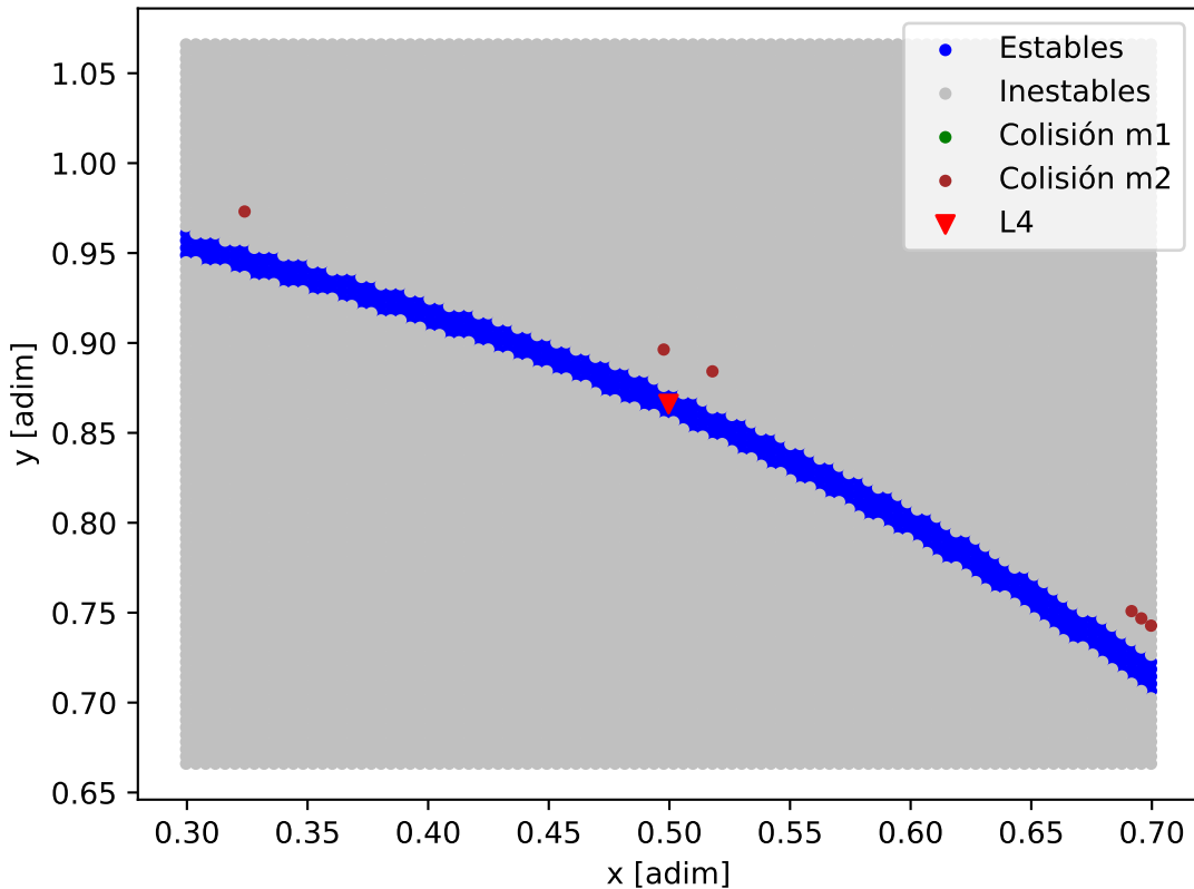
Mapa de estabilidad - HD_34445_HD_34445_g
