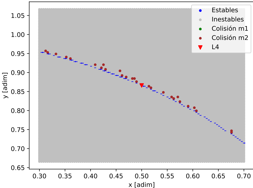
Mapa de estabilidad - HD_63433_HD_63433_d
