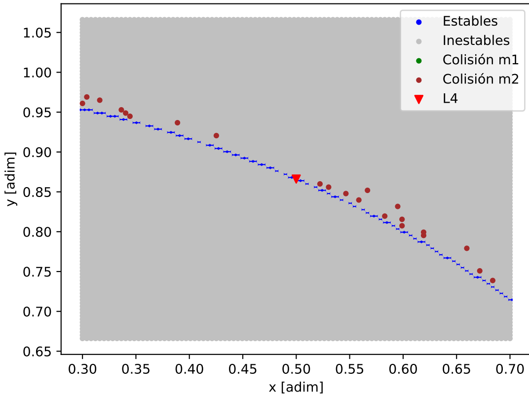
Mapa de estabilidad - HD_93385_HD_93385_b
