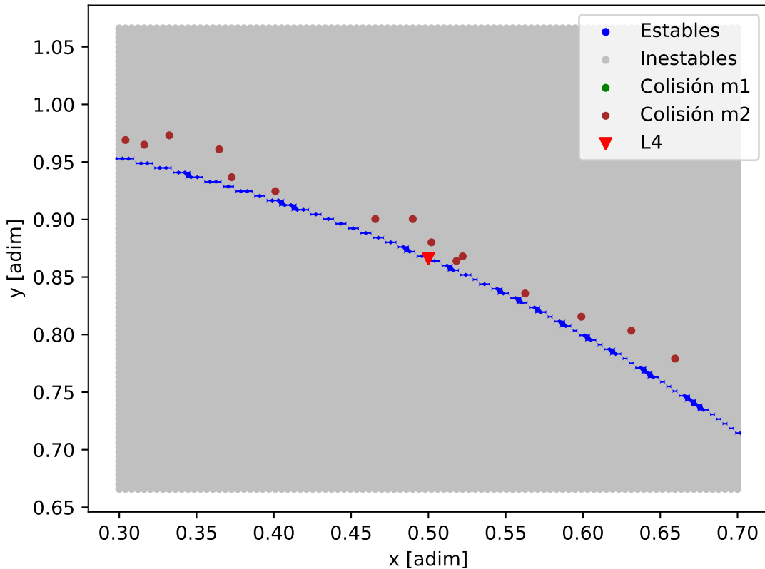
Mapa de estabilidad - HD_93385_HD_93385_d
