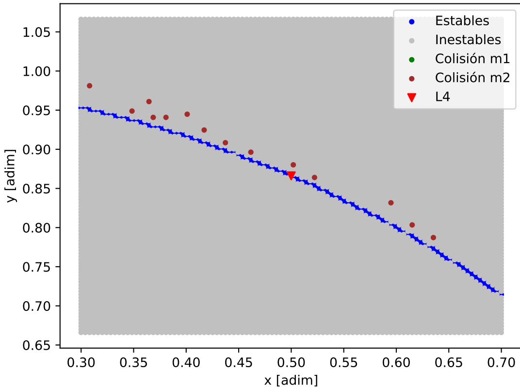
Mapa de estabilidad - HD_96700_HD_96700_d
