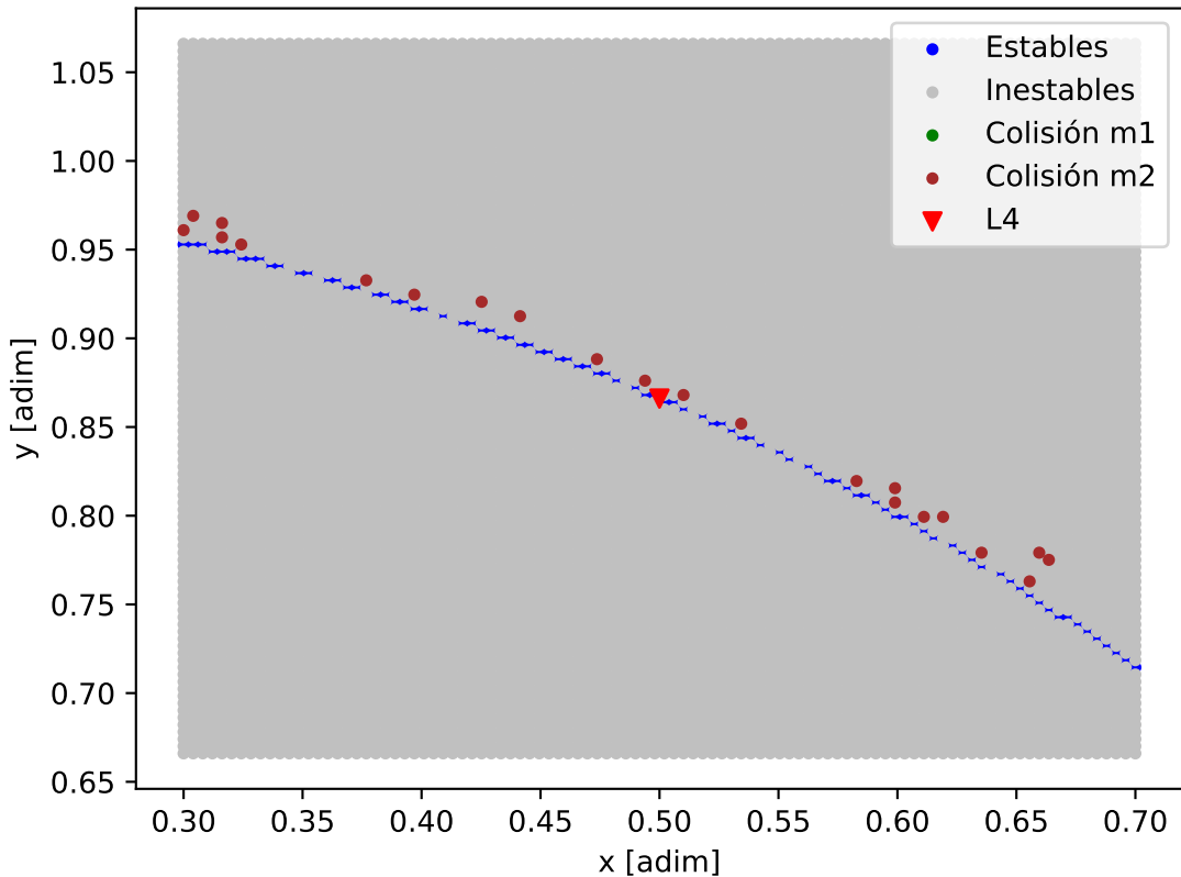
Mapa de estabilidad - K2-138_K2-138_b
