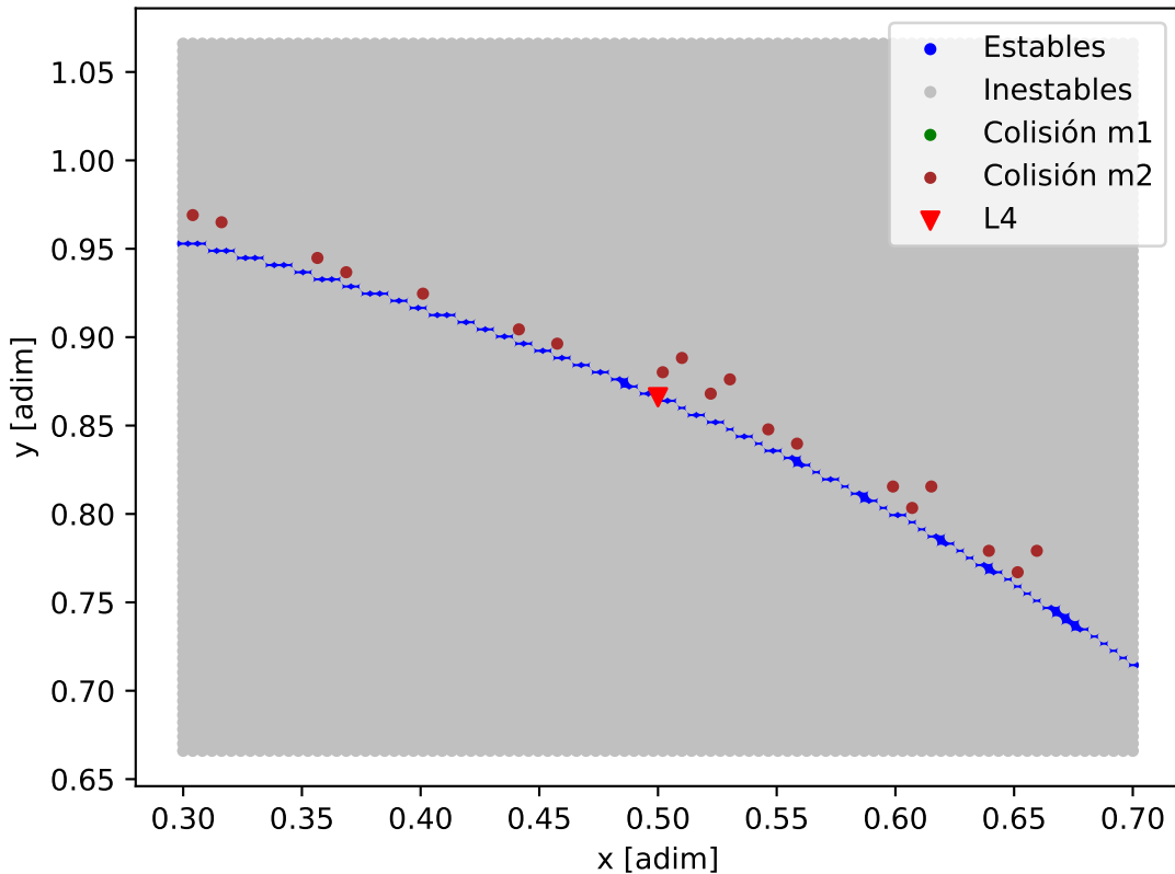
Mapa de estabilidad - K2-138_K2-138_c
