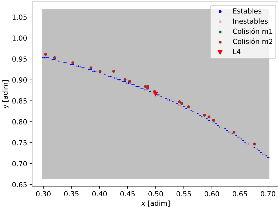
Mapa de estabilidad - K2-138_K2-138_f
