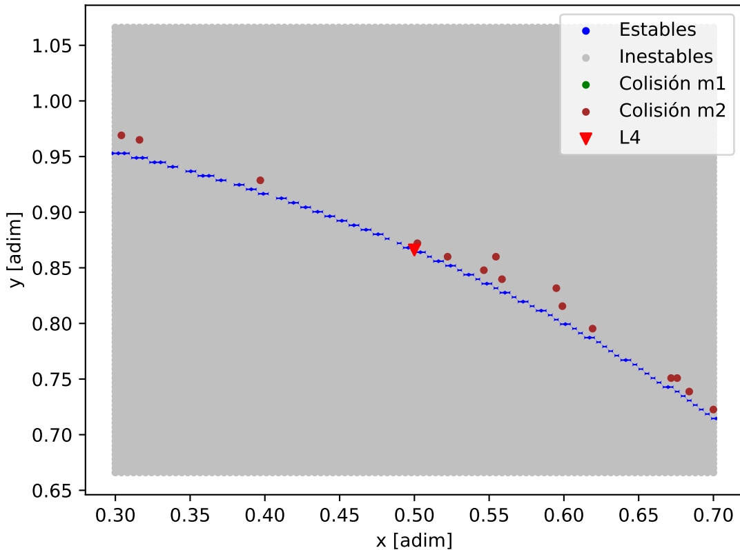
Mapa de estabilidad - K2-138_K2-138_g
