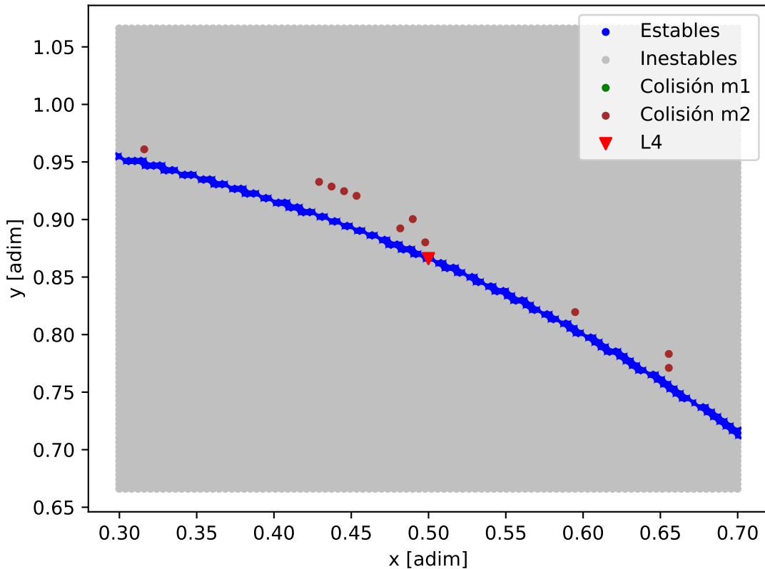
Mapa de estabilidad - K2-157_K2-157_c
