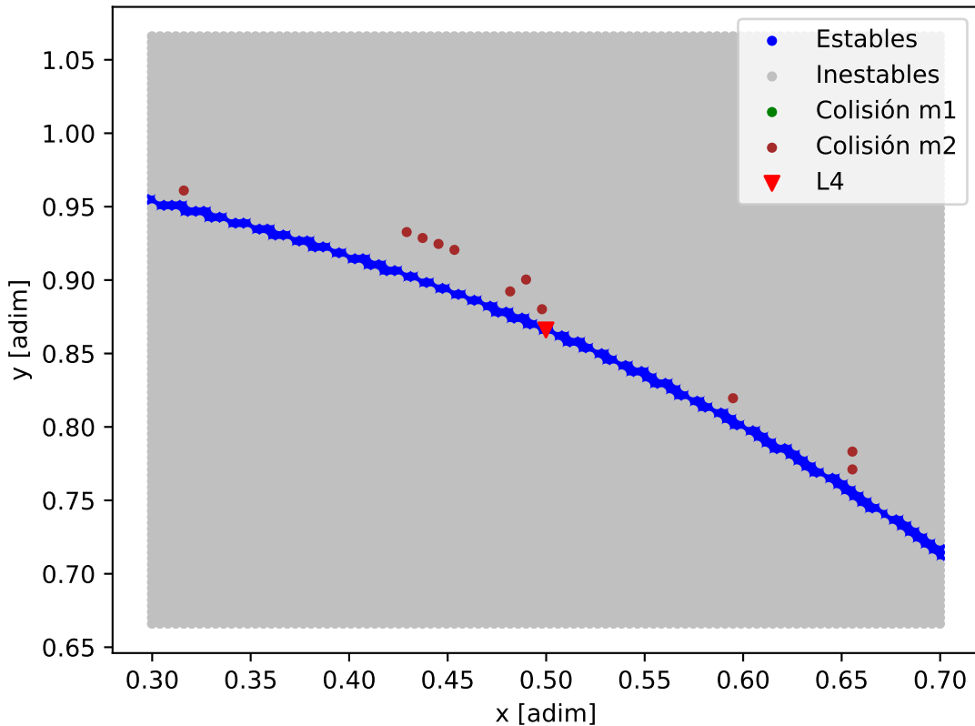
Mapa de estabilidad - K2-19_K2-19_b
