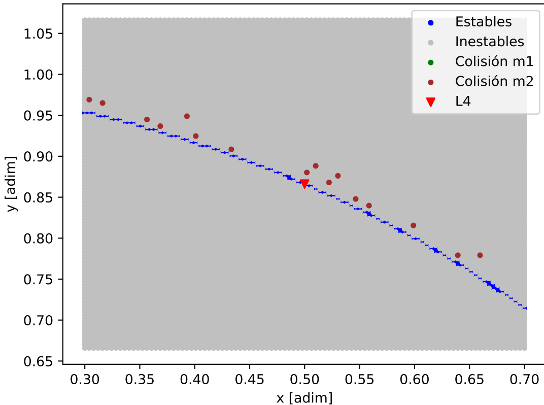
Mapa de estabilidad - K2-19_K2-19_d
