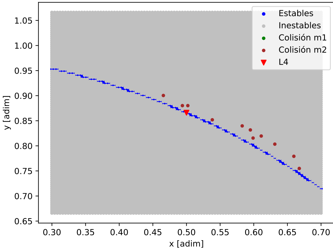
Mapa de estabilidad - K2-32_K2-32_c
