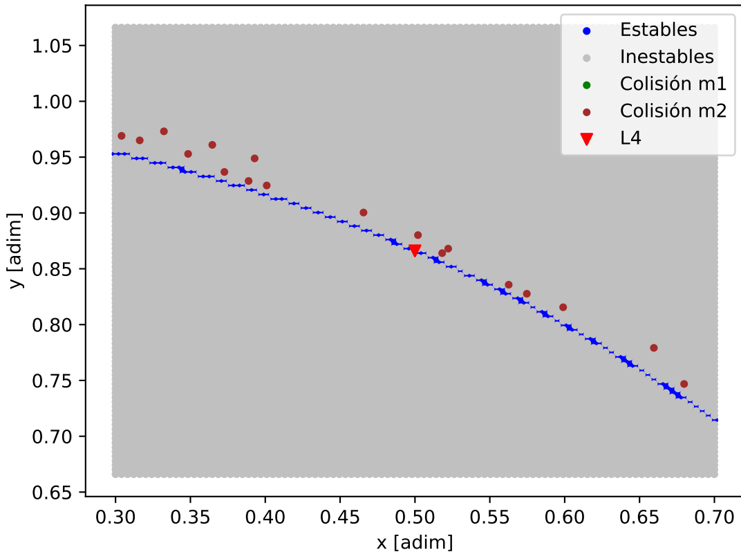
Mapa de estabilidad - K2-32_K2-32_d
