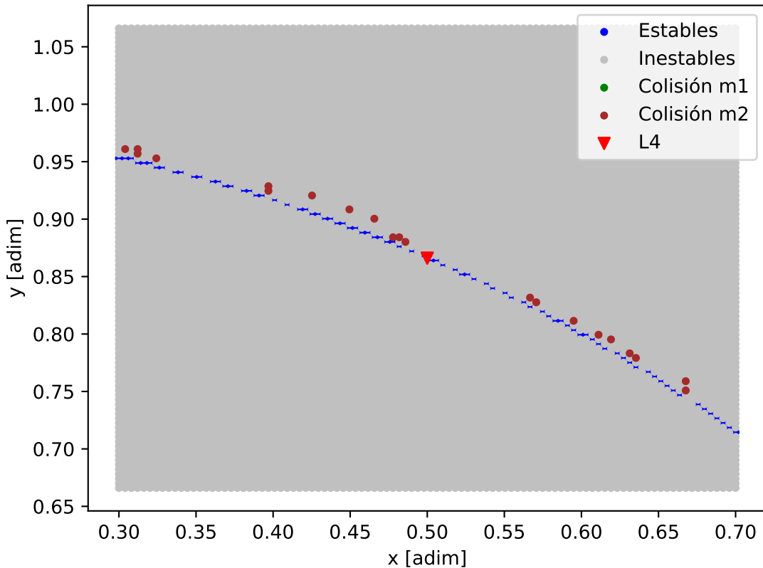
Mapa de estabilidad - K2-32_K2-32_e
