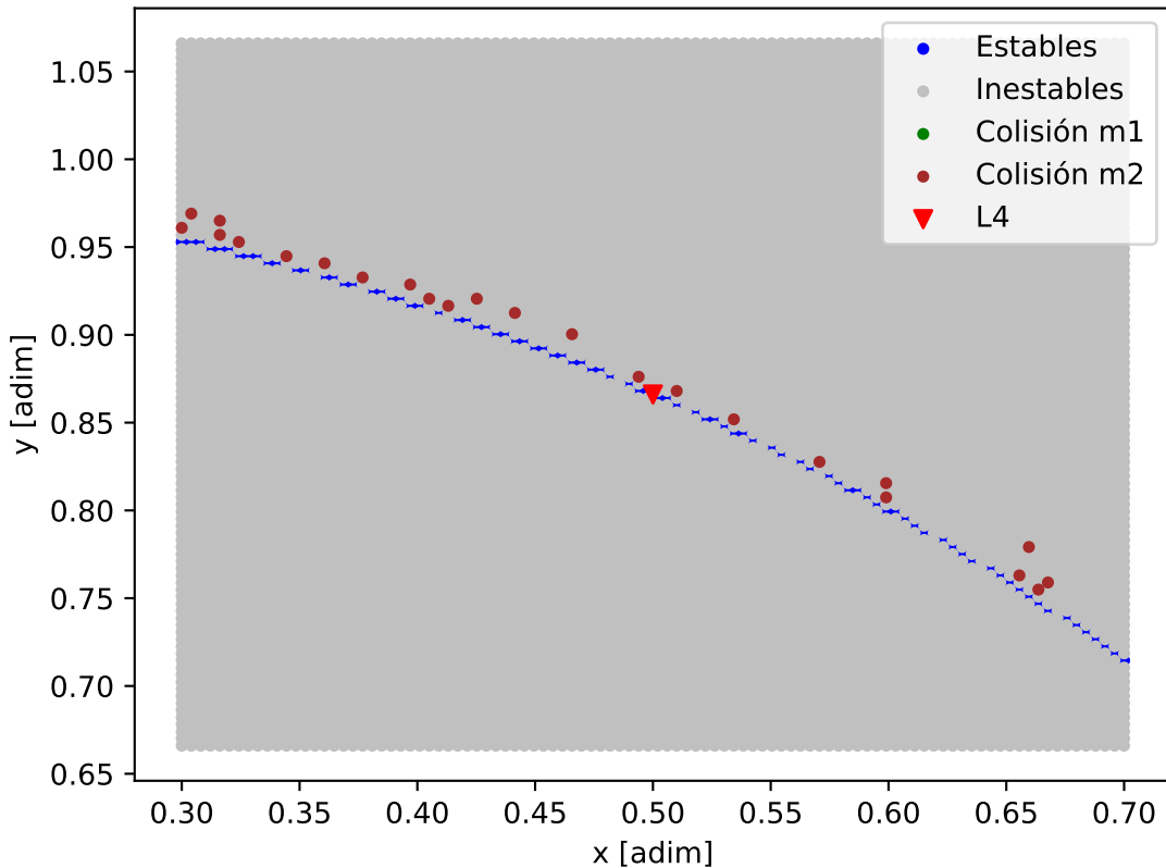
Mapa de estabilidad - K2-37_K2-37_b
