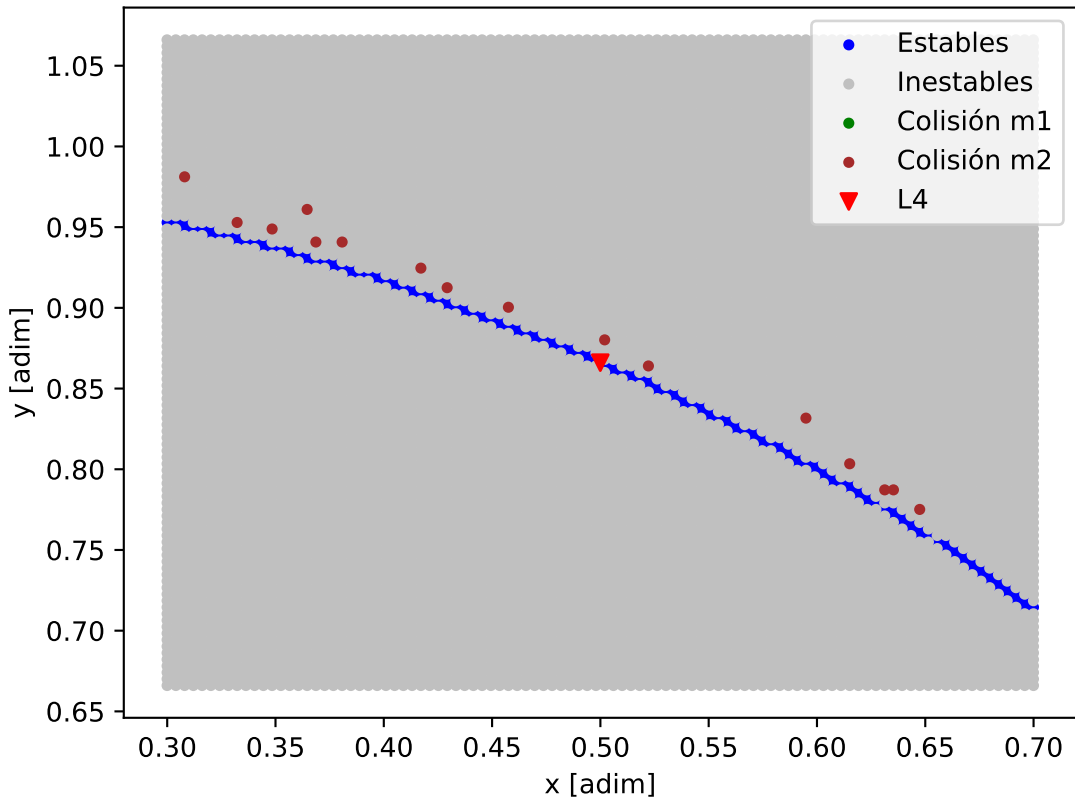
Mapa de estabilidad - K2-37_K2-37_d
