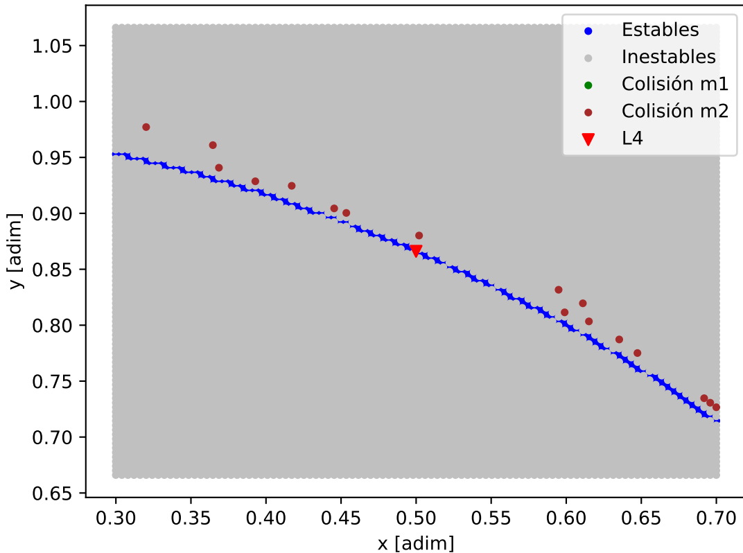
Mapa de estabilidad - Kepler-82_Kepler-82_b
