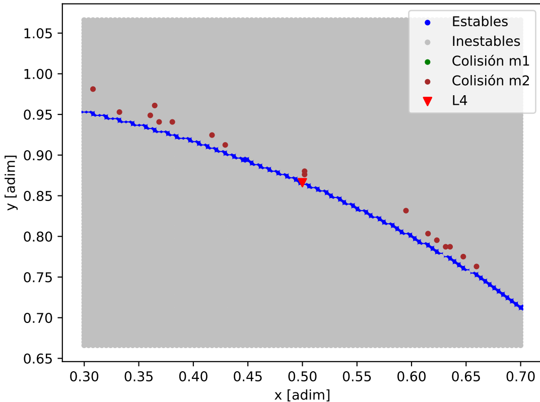
Mapa de estabilidad - Kepler-82_Kepler-82_c
