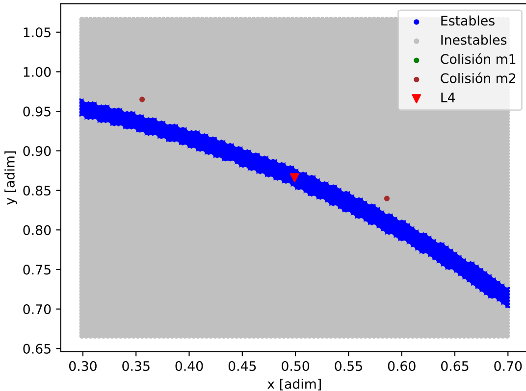
Mapa de estabilidad - Kepler-82_Kepler-82_e
