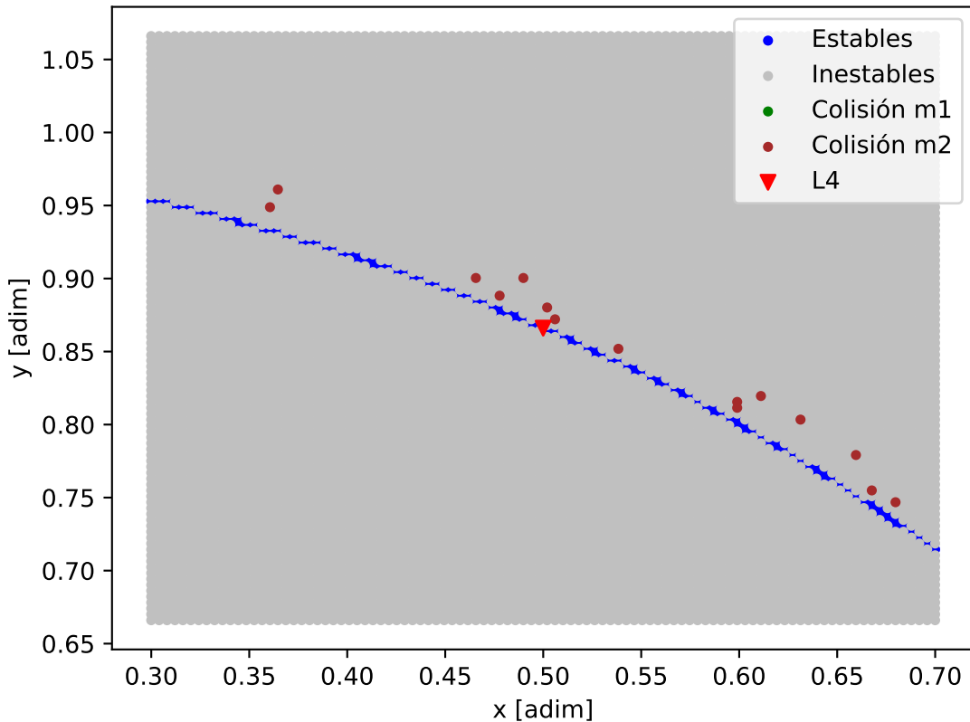
Mapa de estabilidad - TOI-1117_TOI-1117_b
