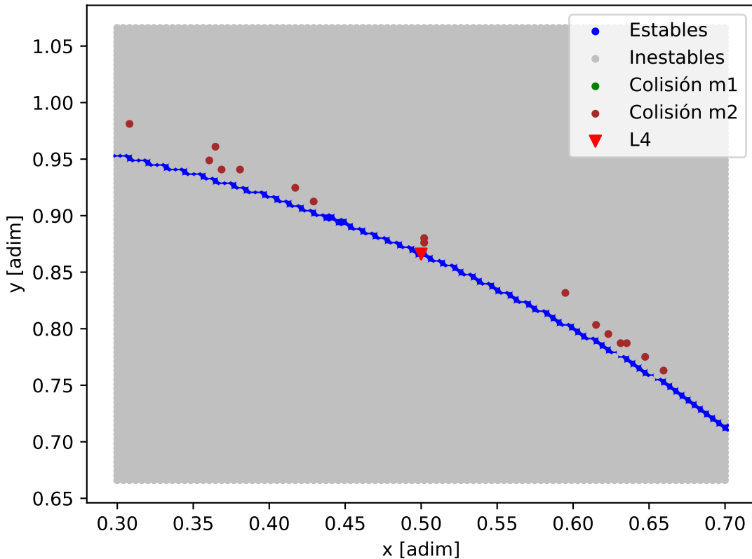
Mapa de estabilidad - TOI-561_TOI-561_e
