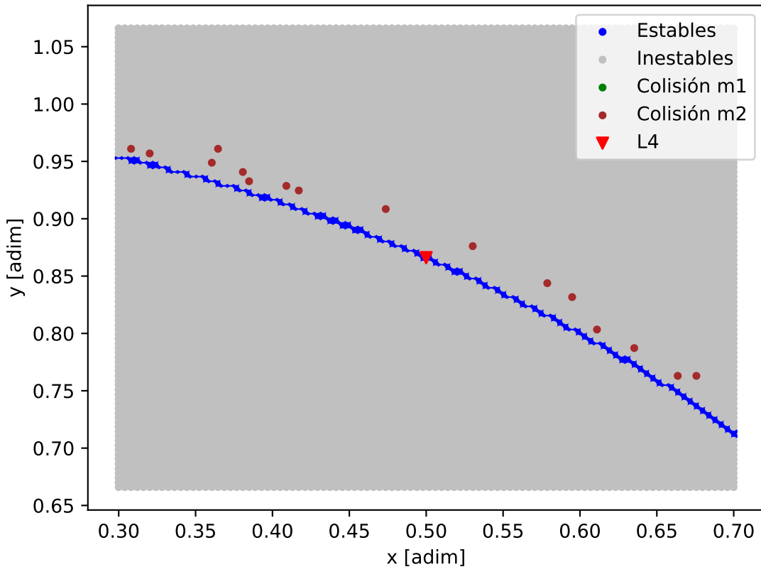
Mapa de estabilidad - TOI-7510_TOI-7510_b
