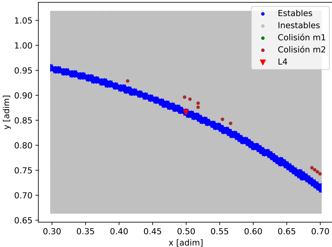
Mapa de estabilidad - TOI-7510_TOI-7510_c
