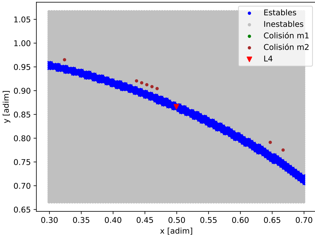
Mapa de estabilidad - TOI-7510_TOI-7510_d
